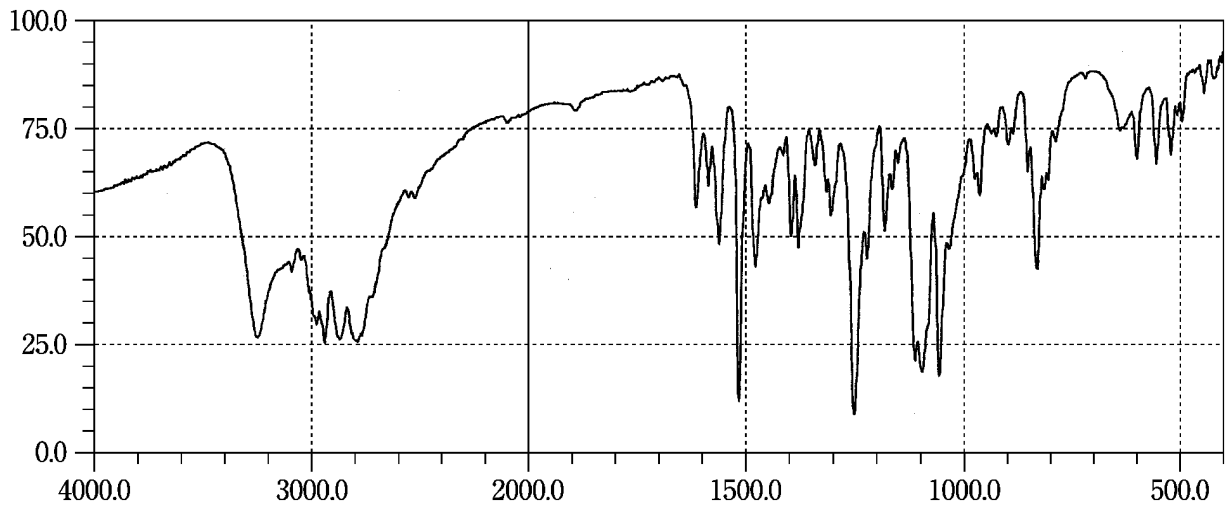
Betaxolol Hydrochloride
