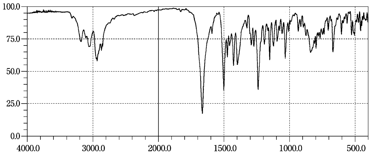
Cilostazol
