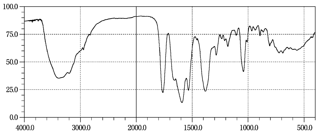
Cefodizime Sodium
