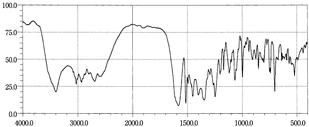
Ifenprodil Tartrate
