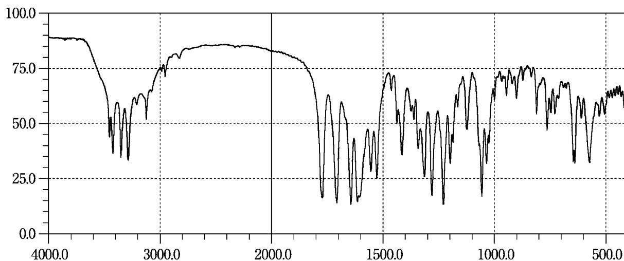
Carumonam Sodium
