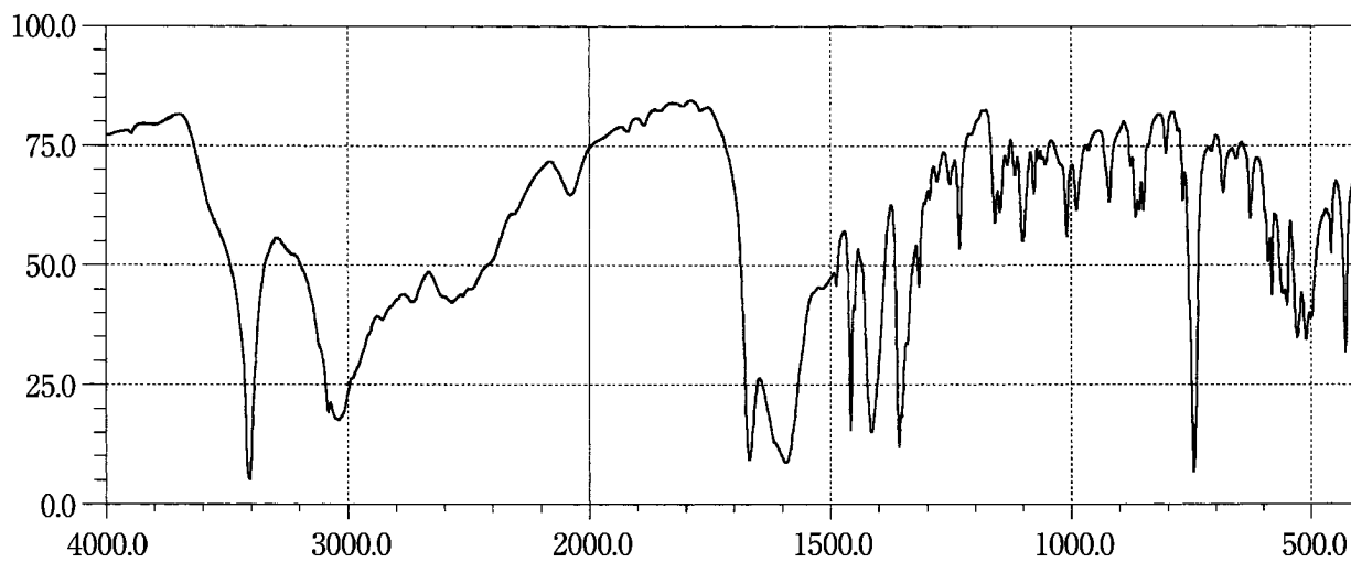
L-Tryptophan
