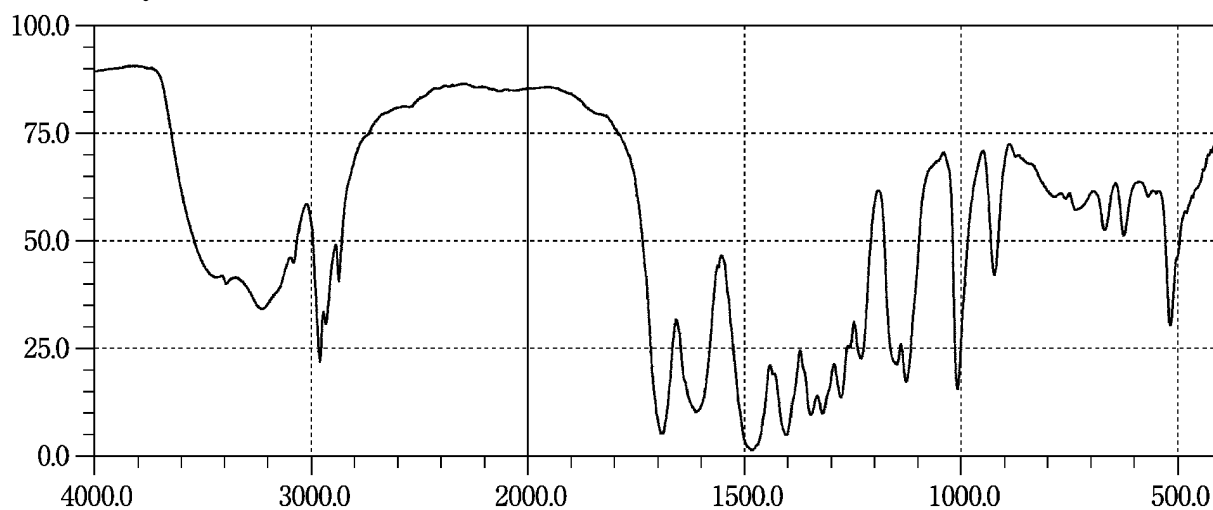
Thiamylal Sodium
