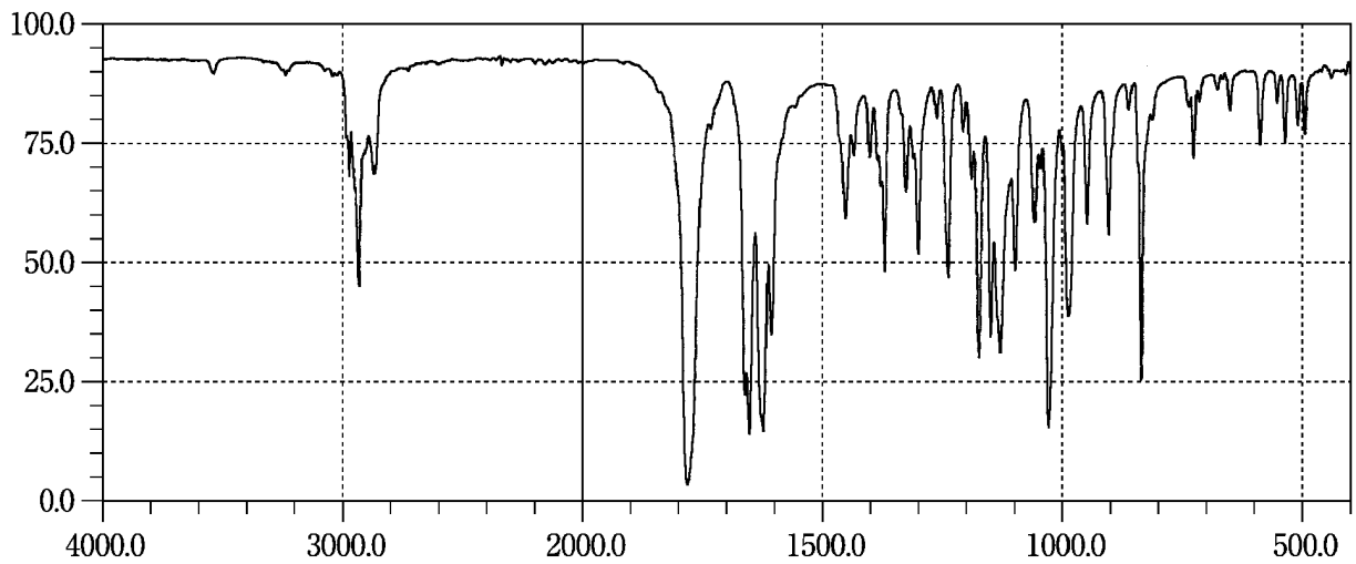
Santonin
