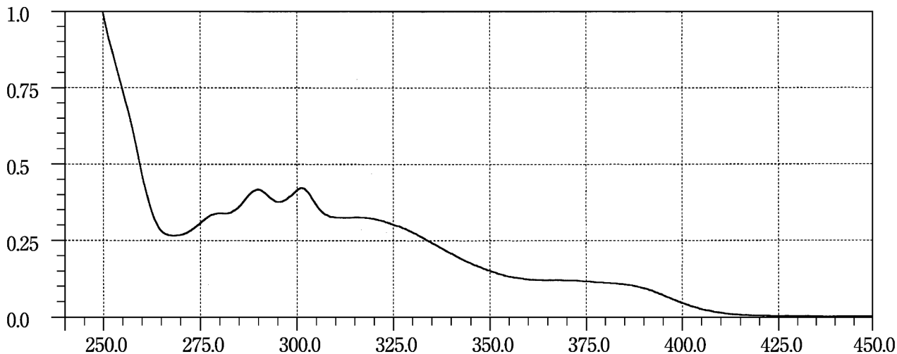
Pyrantel Pamoate
