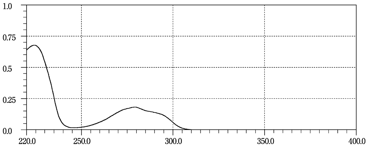
Tamsulosin Hydrochloride
