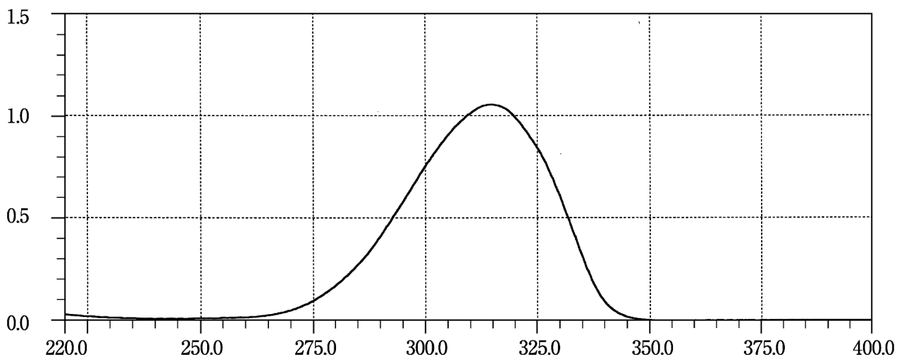
Oxymetholone
