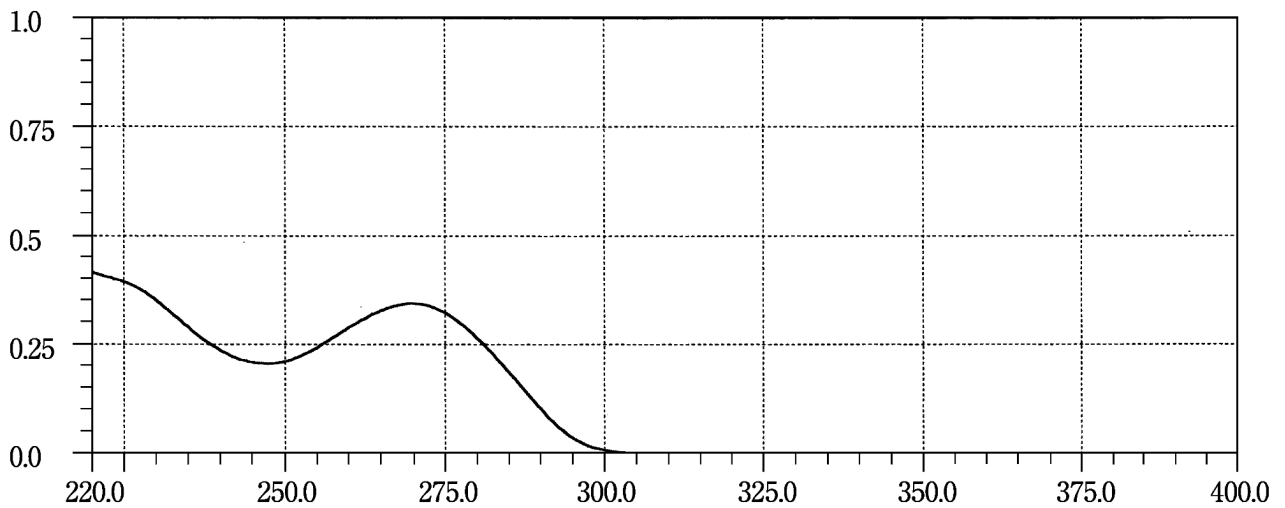
Tegafur
