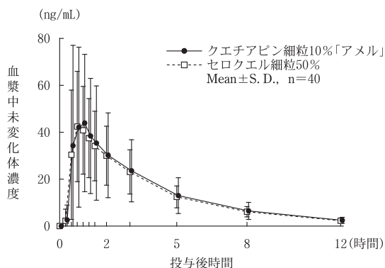
図3 血漿中未変化体濃度（生物学的同等性）
