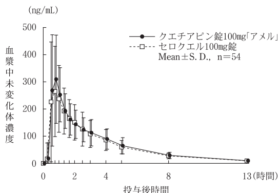
図2 血漿中未変化体濃度（生物学的同等性）
