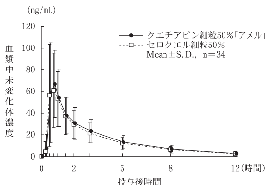
図4 血漿中未変化体濃度（生物学的同等性）
