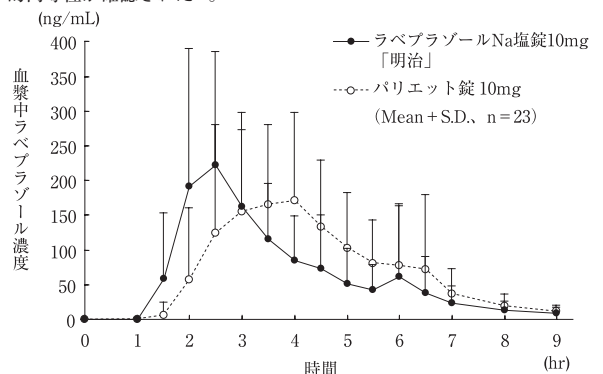
図 10mg錠投与時の血漿中ラベプラゾール濃度推移
