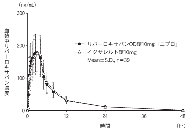
血漿中リバーロキサバン濃度推移 (水あり投与)
