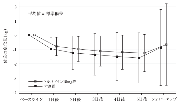
図17-1 体重のベースラインからの変化量
