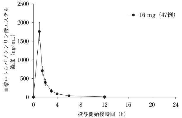
図16-1 健康成人における本剤16mg単回静脈内投与(1時間かけて投与)時の血漿中トルバプタンリン酸エステル濃度推移(平均値±標準偏差)
