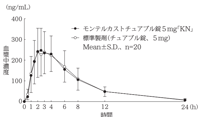
図3 モンテルカストの血漿中濃度推移
