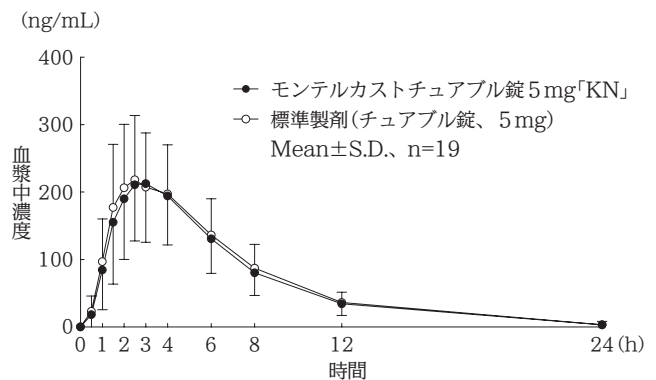
図1 モンテルカストの血漿中濃度推移
