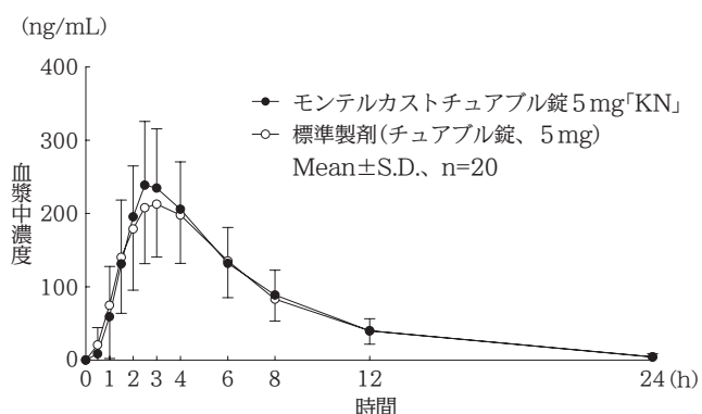
図4 モンテルカストの血漿中濃度推移
