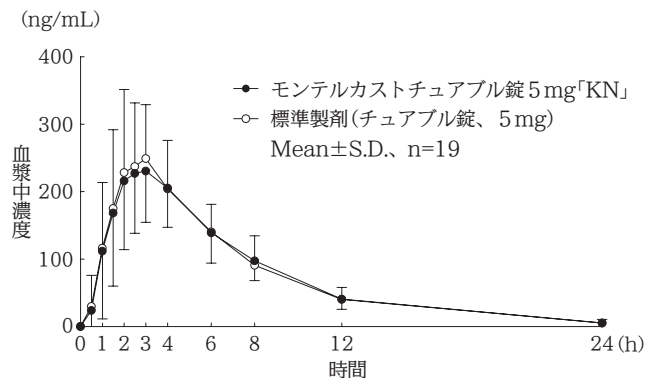
図2 モンテルカストの血漿中濃度推移
