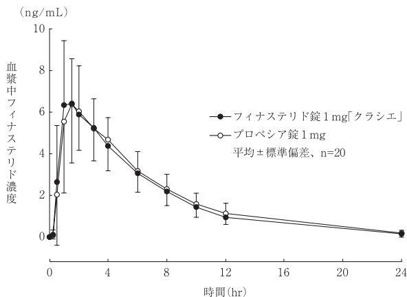
図1 血漿中フィナステリド濃度推移
