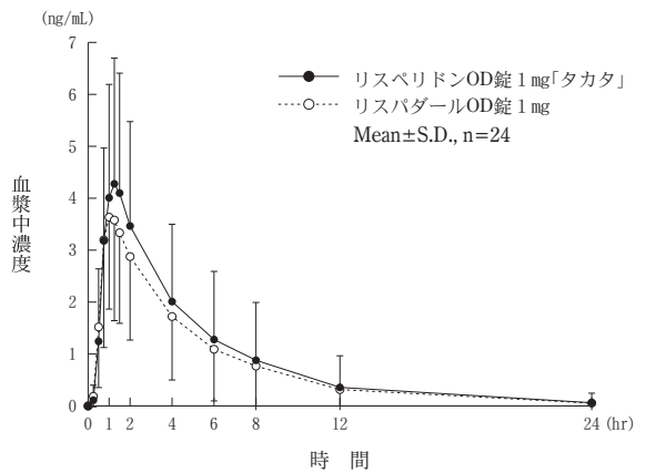
図 16-2 血漿中濃度（OD錠1mg、水で服用）
