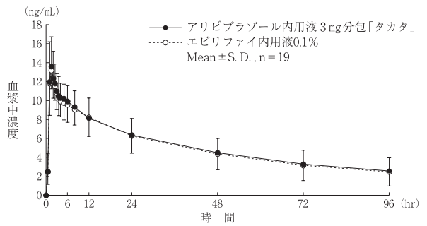
図16-1 血漿中濃度
