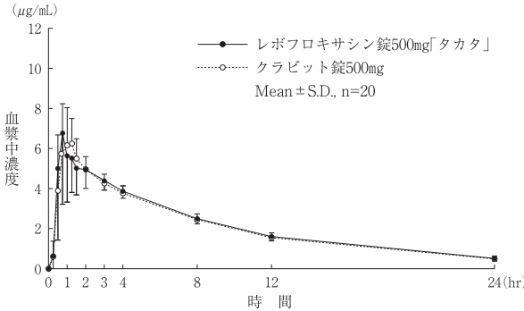
図 16-1 血漿中濃度
