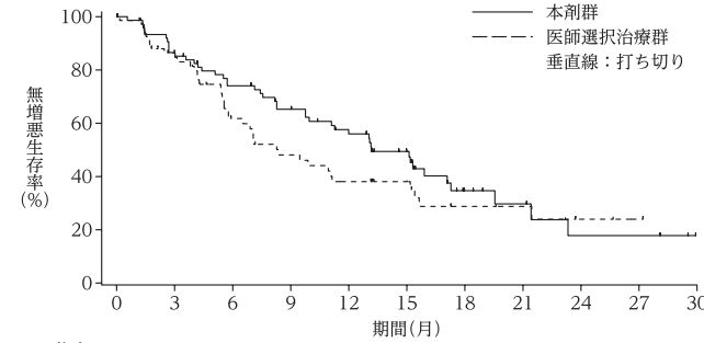
無増悪生存期間のKaplan-Meier曲線(HER2超低発現集団)
