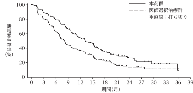
無増悪生存期間のKaplan-Meier曲線(HER2低発現集団)
