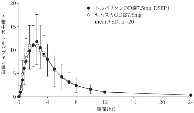
薬物動態パラメータ(R-トルバプタン 絶食時・水あり投与)
