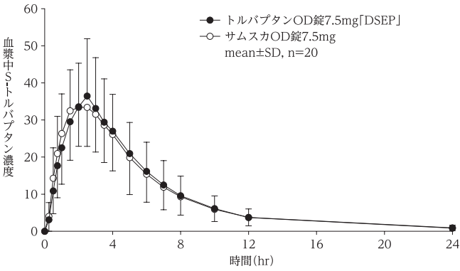
薬物動態パラメータ(S-トルバプタン 絶食時・水あり投与)
