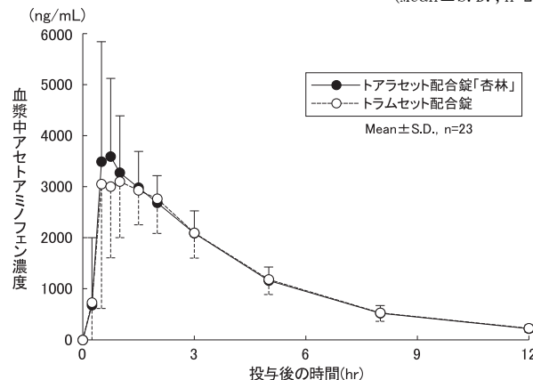
図16-2 血漿中アセトアミノフェン濃度
