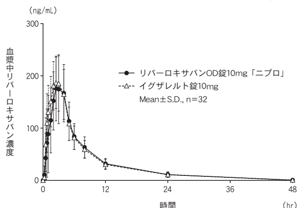
血漿中リバーロキサバン濃度推移（水なし投与）
