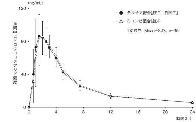
血漿中薬物濃度推移 (ヒドロクロロチアジド)
