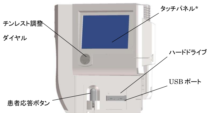
図 1 外観図
