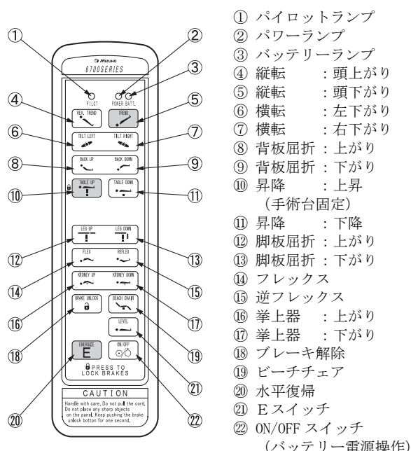
**18-200-20 電動油圧手術台 MOT-6702 (ASIA)
