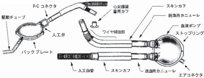
図1 構成部品及び名称
