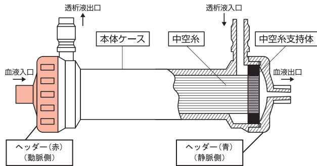
図1 外観と構造
