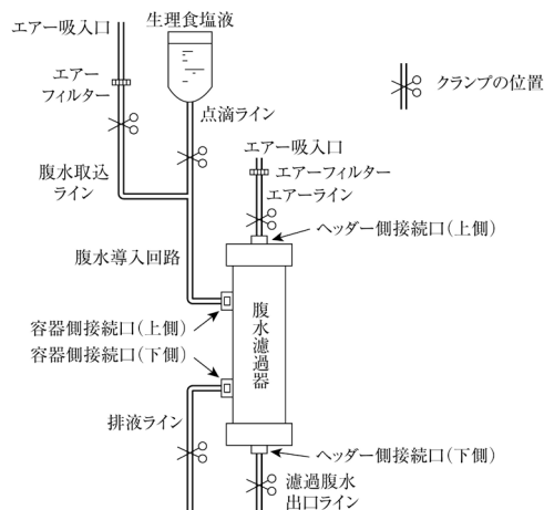
図 4 外圧濾過法・落差式の回路図
