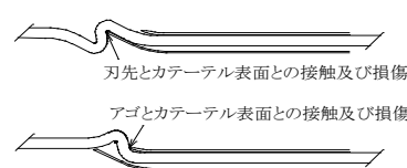
図4. 硬麻針とカテーテルの接触及び損傷の例
