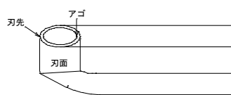
図5. 硬麻針先端部の名称
