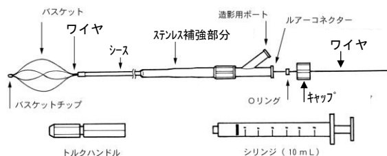
図1: クラッシャーカテーテル本体及び付属品
