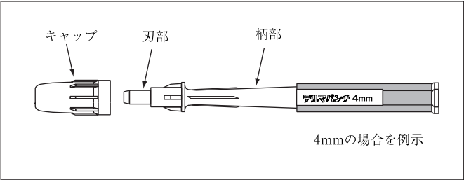
デルマパンチの形状・構造
