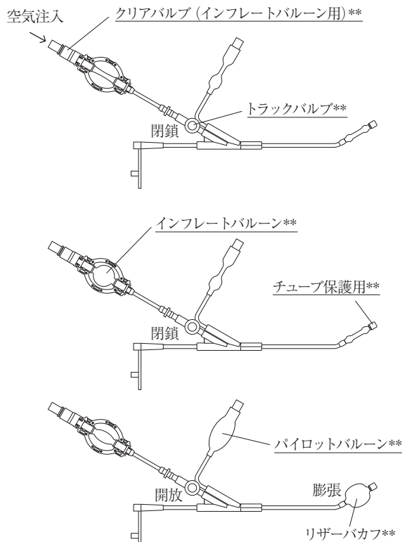
(図3) クーデック気管支ブロッカーチューブ(タイプB) 作動・動作原理図**
