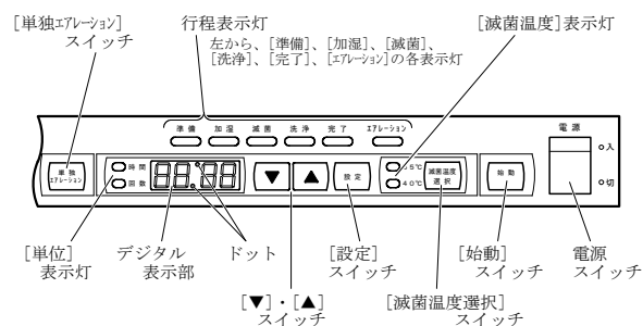
操作パネル
