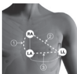
①オルタネイト(リードI)、②セカンダリ(リードII)、③ブライマリ(リードIII) RA—右腕、LA—左腕、LL—左脚
