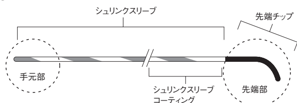
＜図は先端チップ形状がアングルのものを示す＞
