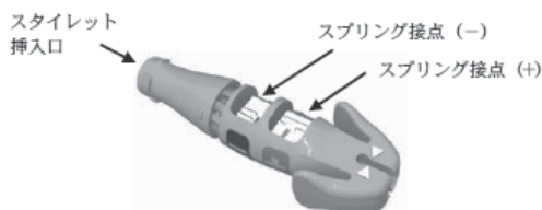
図1: EZ-4コネクタツール
