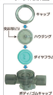
【図5：呼吸弁分解図】
