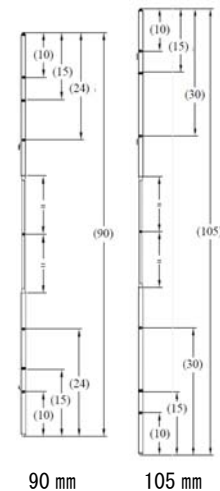
図2 寸法図（正面）
