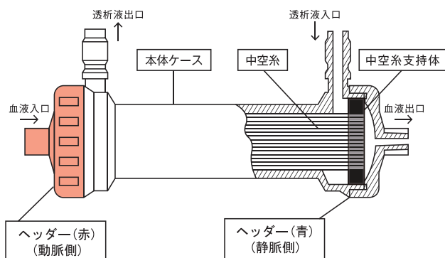
図1 本品の外観と構造
