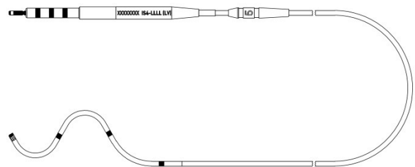
Sentus ProMRI OTW QP L-85/49
