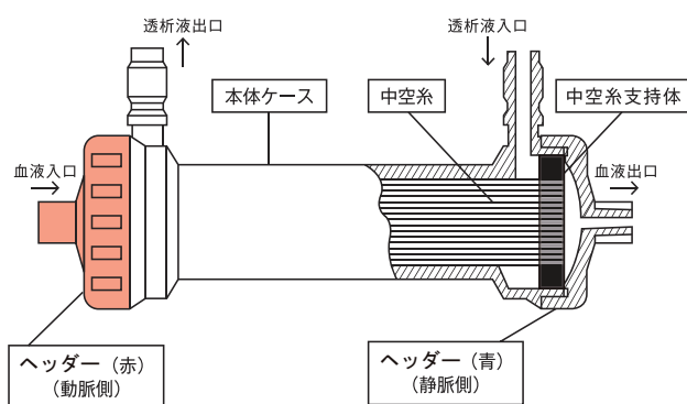
図1 外観と構造
