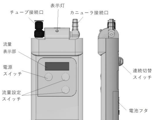
各部の名称及び機能
