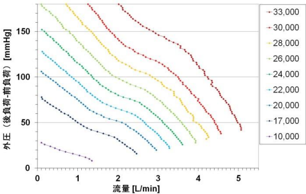
IMPELLA 5.0 の流量特性
