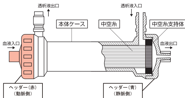
図1 外観と構造
