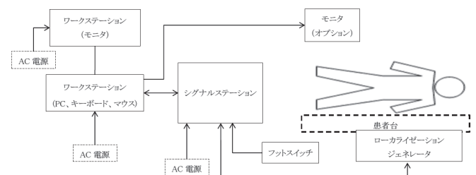
図1 システム接続例
