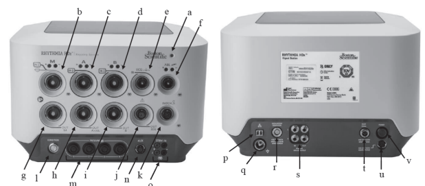
図2 シグナルステーション各接続部
