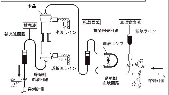
図1 治療前準備及びプライミング時の回路への接続例
