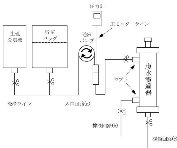
図 2 外圧濾過法(ポンプ式)の回路図
