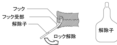
図. クランプのロック解除方法
