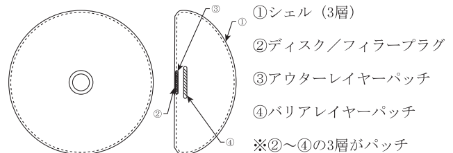
図1 全体図
