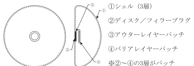
図1 全体図
