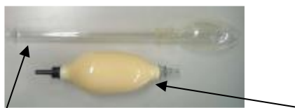
①バルーン トロッカー ディスポーザブル シャフト ②エアポンプ
