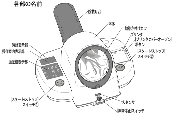
機器構成一覧
