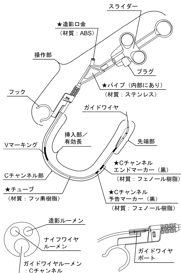
Cチャンネル部断面図
