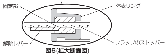
図6(拡大断面図)
