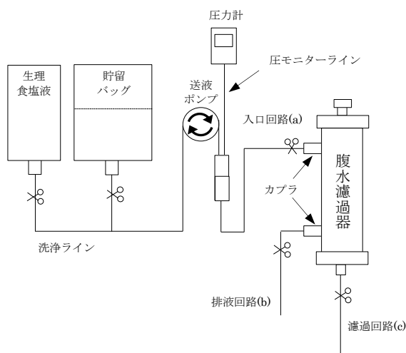
図 2 陽圧ポンプ式外圧濾過法の回路図
