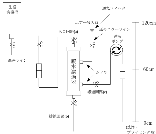
図 3 陰圧ポンプ式内圧濾過法の回路図 (リークチェック、洗浄・プライミング工程時)
