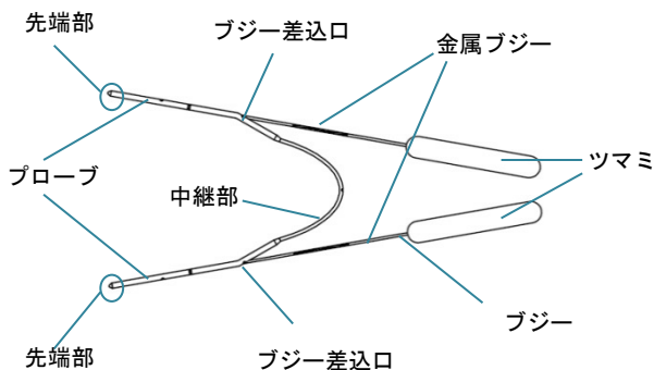
図 1 外観図
